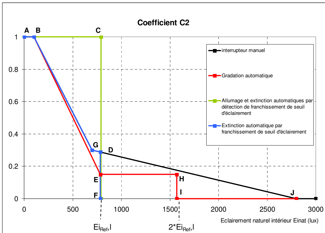
Figure 75 : Courbes donnant les valeurs de C2 selon l'éclairage naturel intérieur et le mode de gestion des apports de lumière naturelle. Exemple pour un éclairage intérieur E_{i,Ref,l} supérieur à 700 lux.
