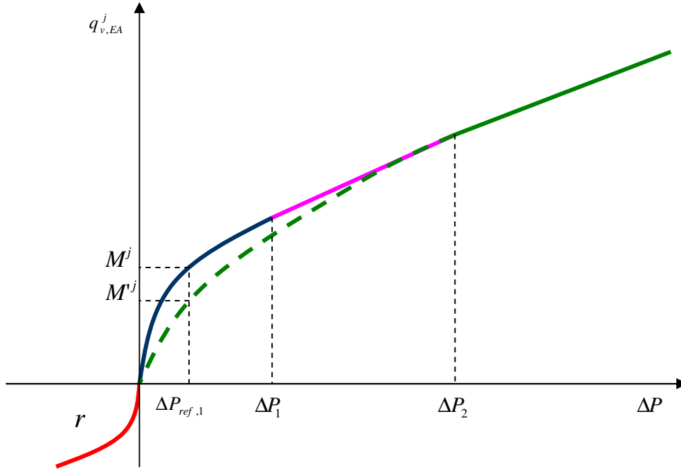
Figure 14 : Courbe caractéristique d'un entrée. On montre l'ensemble des entrées utilisateurs qui peuvent être ajustées afin d'obtenir une entrée d'air fixe ou bien pour obtenir un comportement autoréglable anti-retour.
