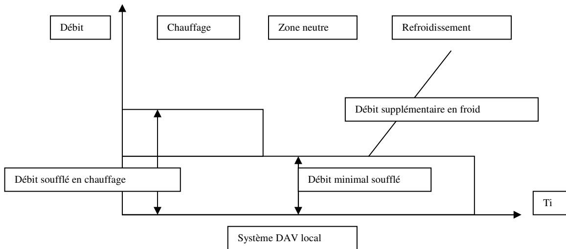
Figure 66 : Principe de fonctionnement d'une unité terminale DAV
