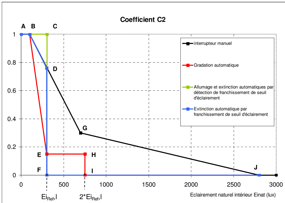
Figure 74 : Courbes donnant les valeurs de C2 selon l'éclairage naturel intérieur et le mode de gestion des apports de lumière naturelle. Exemple pour un éclairage intérieur E_{i,Ref,l} inférieur à 700 lux.
