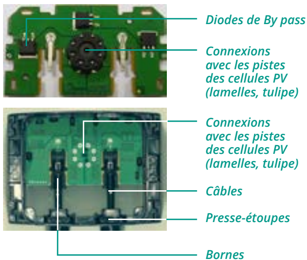
Boîte de jonction avec connecteur central à huit pôles – Source : [7]
