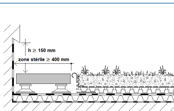
FIGURE 6 RELEVÉ AVEC ZONE STÉRILE TRAITÉE AVEC DALLES SUR PLOTS
