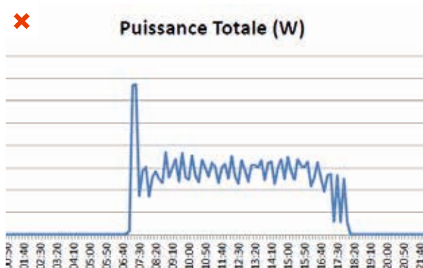
Sur ce site, le groupe froid est dimensionné pour 102 kWf/41 kWe. En pratique, les instrumentations ont montré des puissances réelles nettement inférieures : de l'ordre de 15 à 20 kWe. ©AQC
