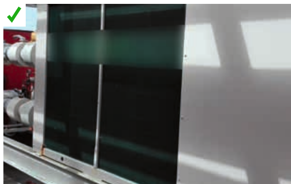
Un protocole de nettoyage a été mis en place dans le cadre d'une maintenance préventive. L'échangeur est rincé à l'eau claire 1 fois par mois et un traitement époxy est appliqué tous les ans, voire tous les semestres pour les sites les plus exposés.
