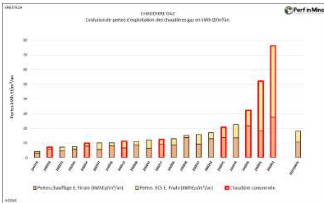
Figure 147 : Histogramme des pertes liées aux rendements de génération.
