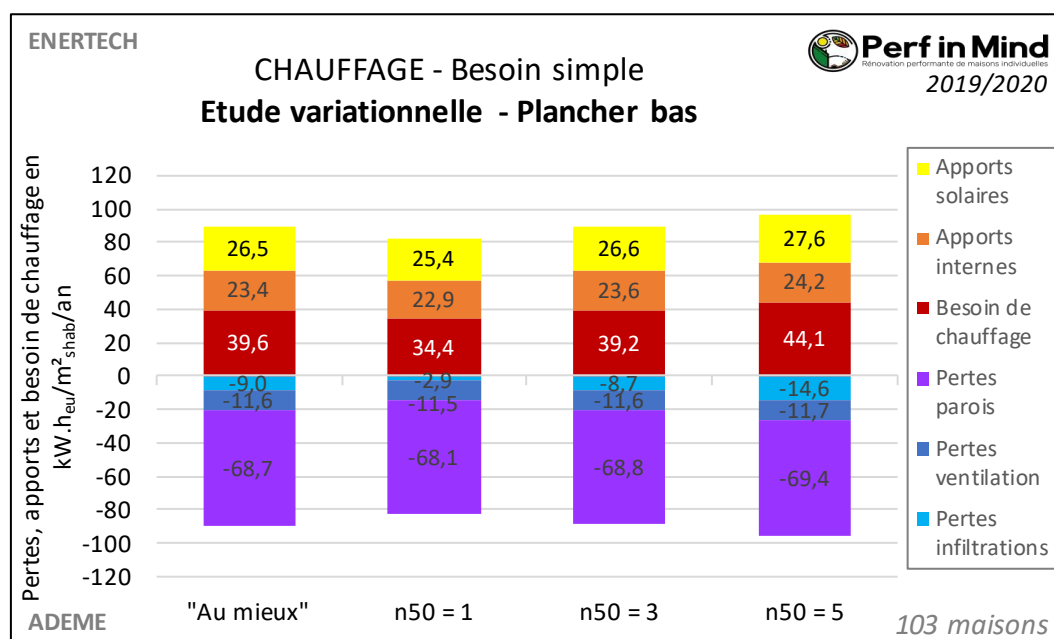
Figure 158 : Graphique du bilan de besoin de chauffage moyens, étude variationnelle en forçant la performance d'étanchéité à l'air à n_{50} = 1 \text{ vol/h} , 3 \text{ vol/h} et 5 \text{ vol/h} .
