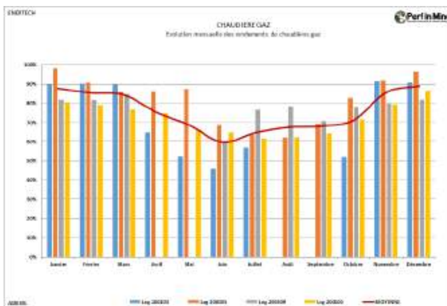
Figure 146 : saisonnalité des rendements de génération.
