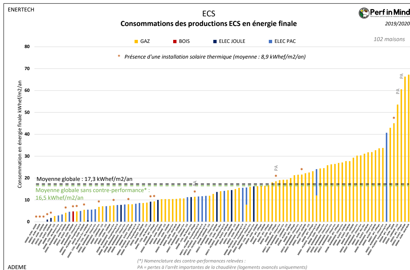
Figure 163 : Consommations d'ECS des projets en énergie finale.
