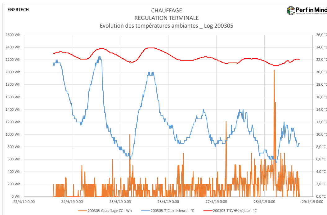
Figure 133 : Graphique d'analyse de la régulation terminale : mauvaise régulation malgré la présence d'un thermostat.
