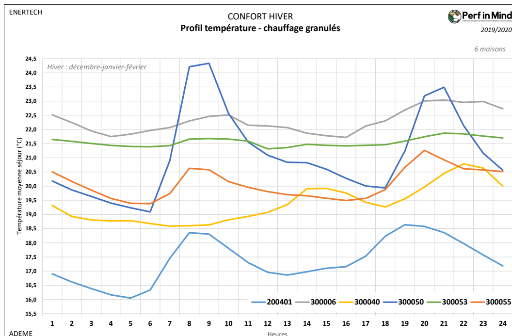
Figure 203 : Graphique des profils de température moyenne sur une journée pour les 6 maisons chauffées avec un poêle à granulés.
