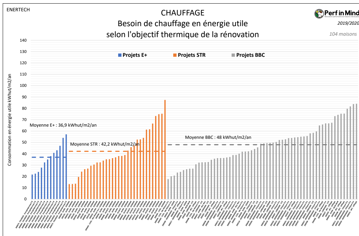
Figure 123 : Besoins de chauffage des logements tirés de la mesure, par type d'objectif thermique.
