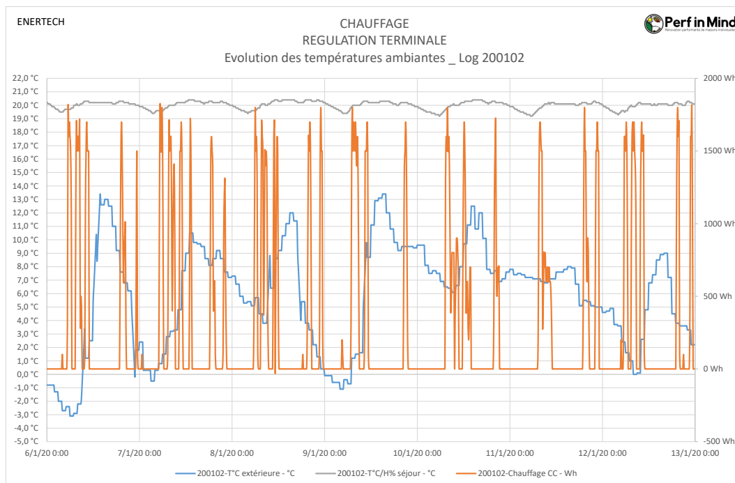
Figure 132 : Graphique d'analyse de la régulation terminale : bon fonctionnement (thermostat).
