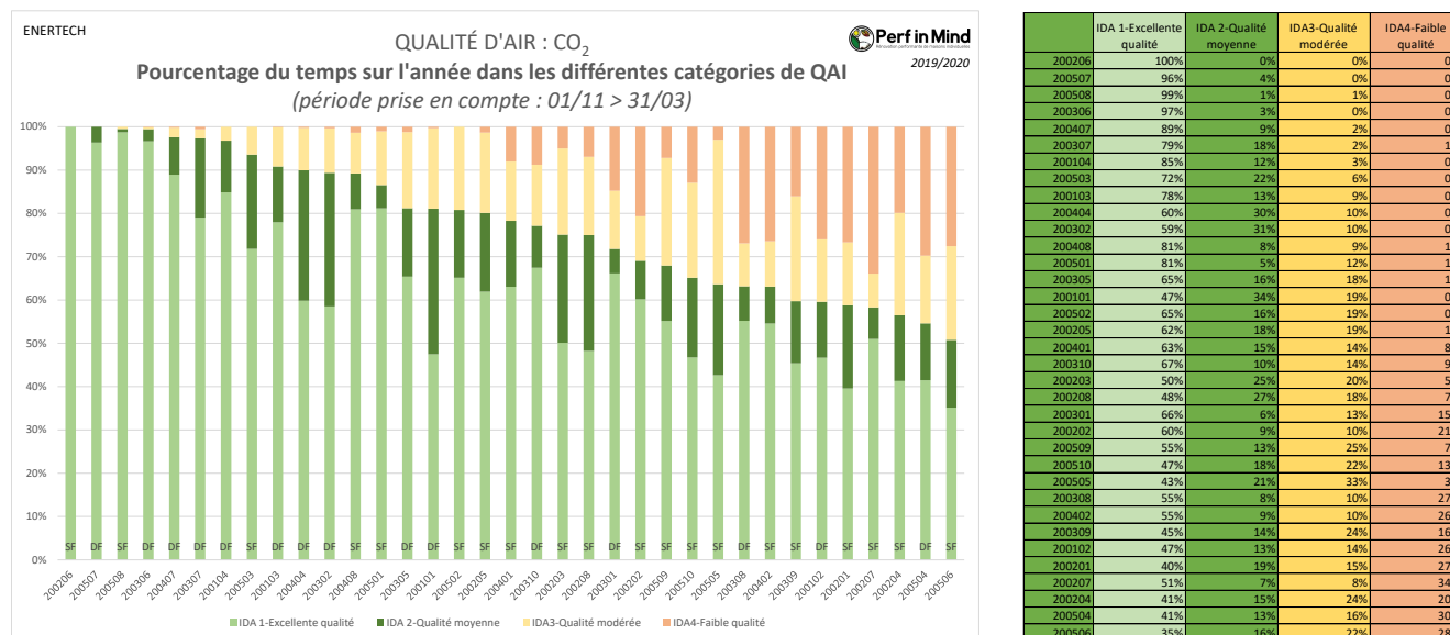
Figure 217 : Pourcentage du temps sur l'année dans les différentes catégories de QAI du 01/11 au 31/03
