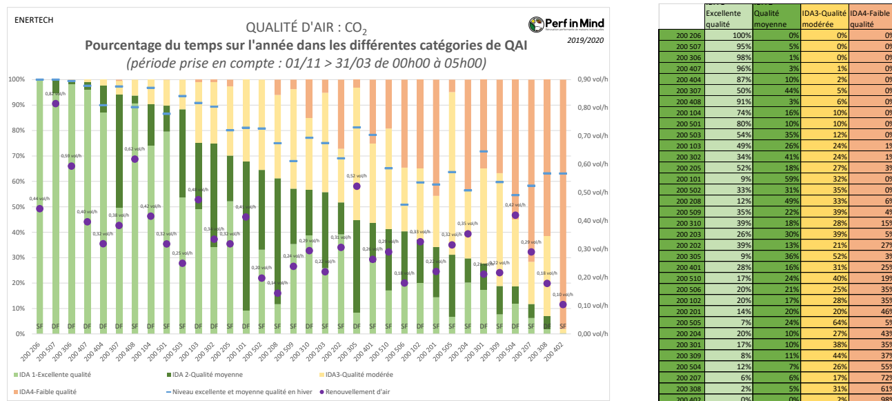
Figure 218 : Qualité d'air – Pourcentage du temps sur l'année dans les différentes catégories de QAI du 01/11 au 31/03 de 00h00 à 05h00
