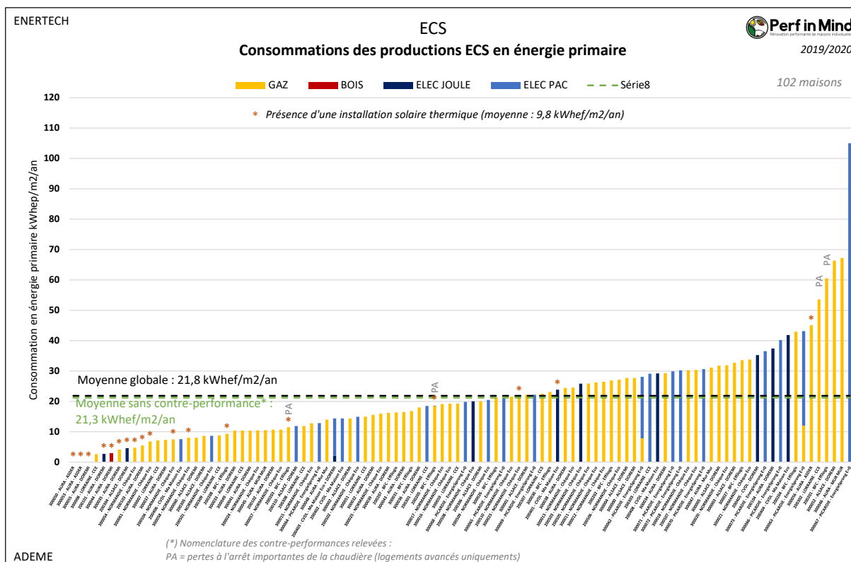
Figure 164 : Consommations d'ECS des projets en énergie primaire.
