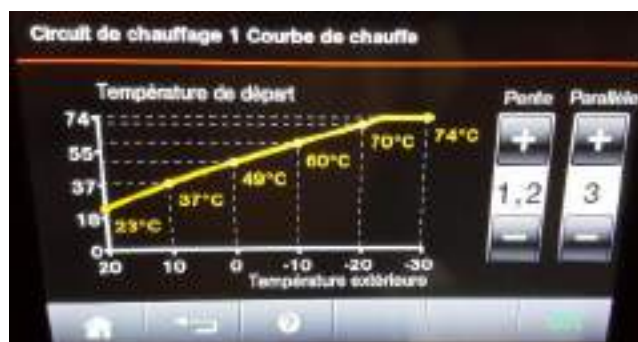
Figure 140 : Illustration : exemple de programmation de la loi d'eau sur une chaudière.
