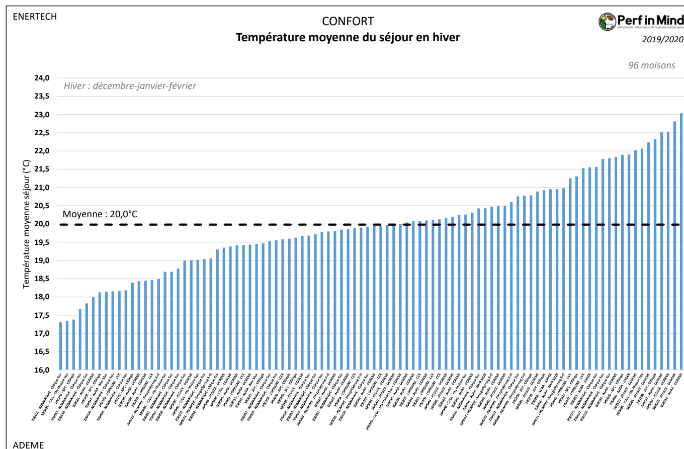
Figure 196 : Graphique des températures moyennes dans le séjour en hiver.
