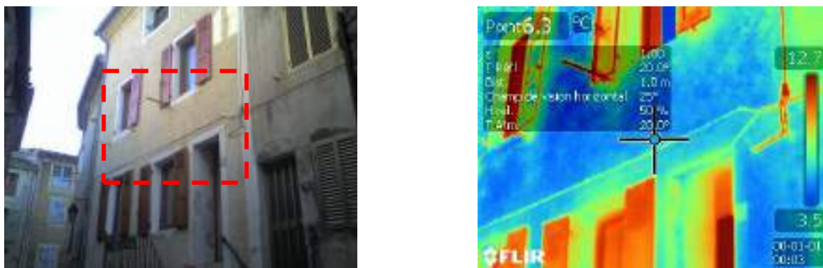
Figure 79 : Thermogramme extérieur de mur isolé par l'intérieur, au niveau du plancher intermédiaire bois.
