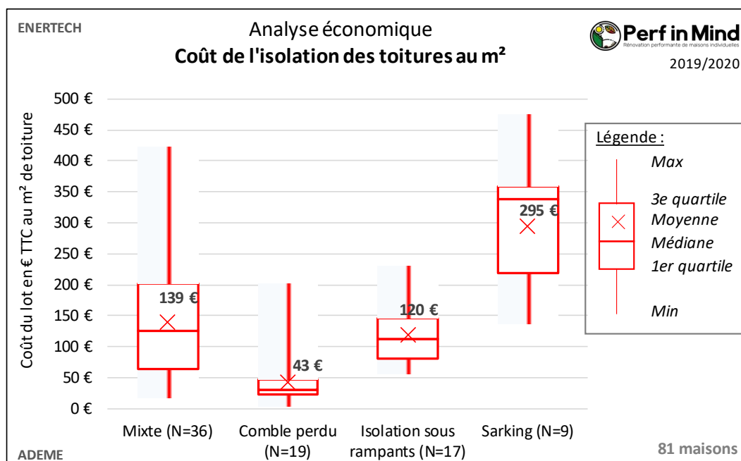
Figure 238 : Graphique des coûts d'isolation des toitures, rapporté à la surface de toiture (selon étude thermique).
