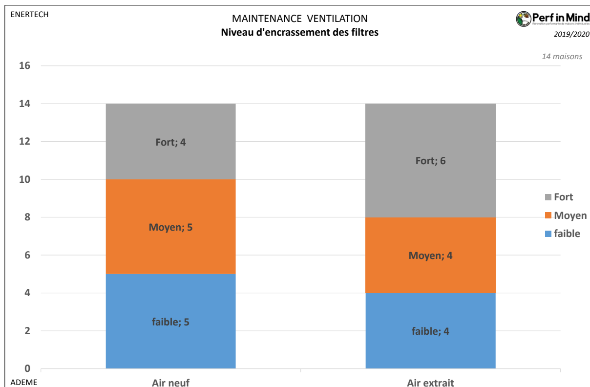
Figure 29 : Graphique du niveau d'encrassement des filtres des VMC double flux lors de l'instrumentation les maisons en suivi « avancé ».
