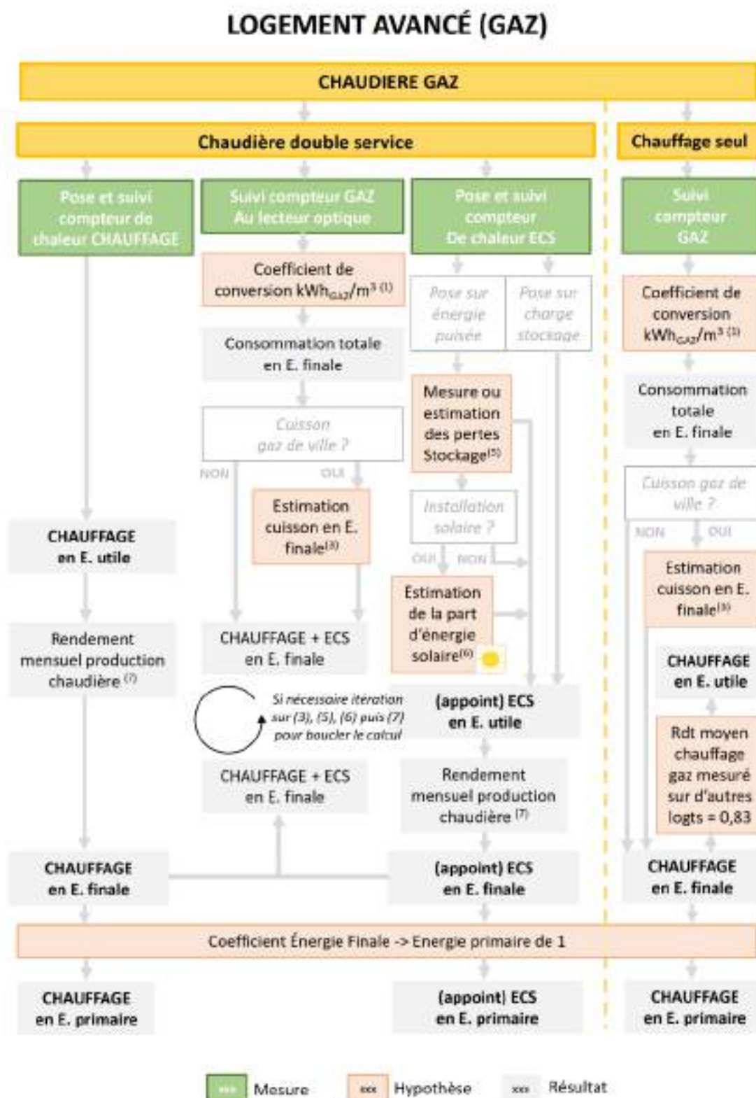
Figure 252 : Post-traitement de la mesure - logement avancé en chauffage gaz.
