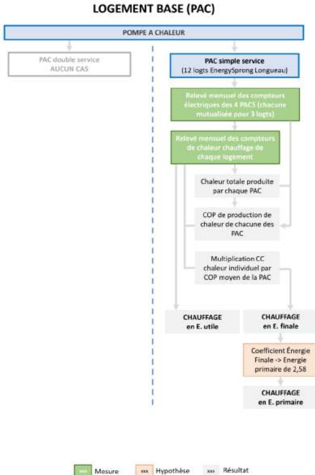
Figure 255 : Post-traitement de la mesure - logement base avec chauffage par pompe à chaleur.
