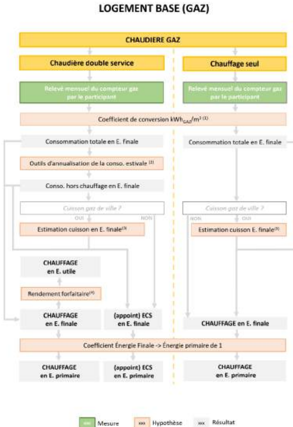
Figure 251 : Post-traitement de la mesure - logement base en chauffage gaz.
