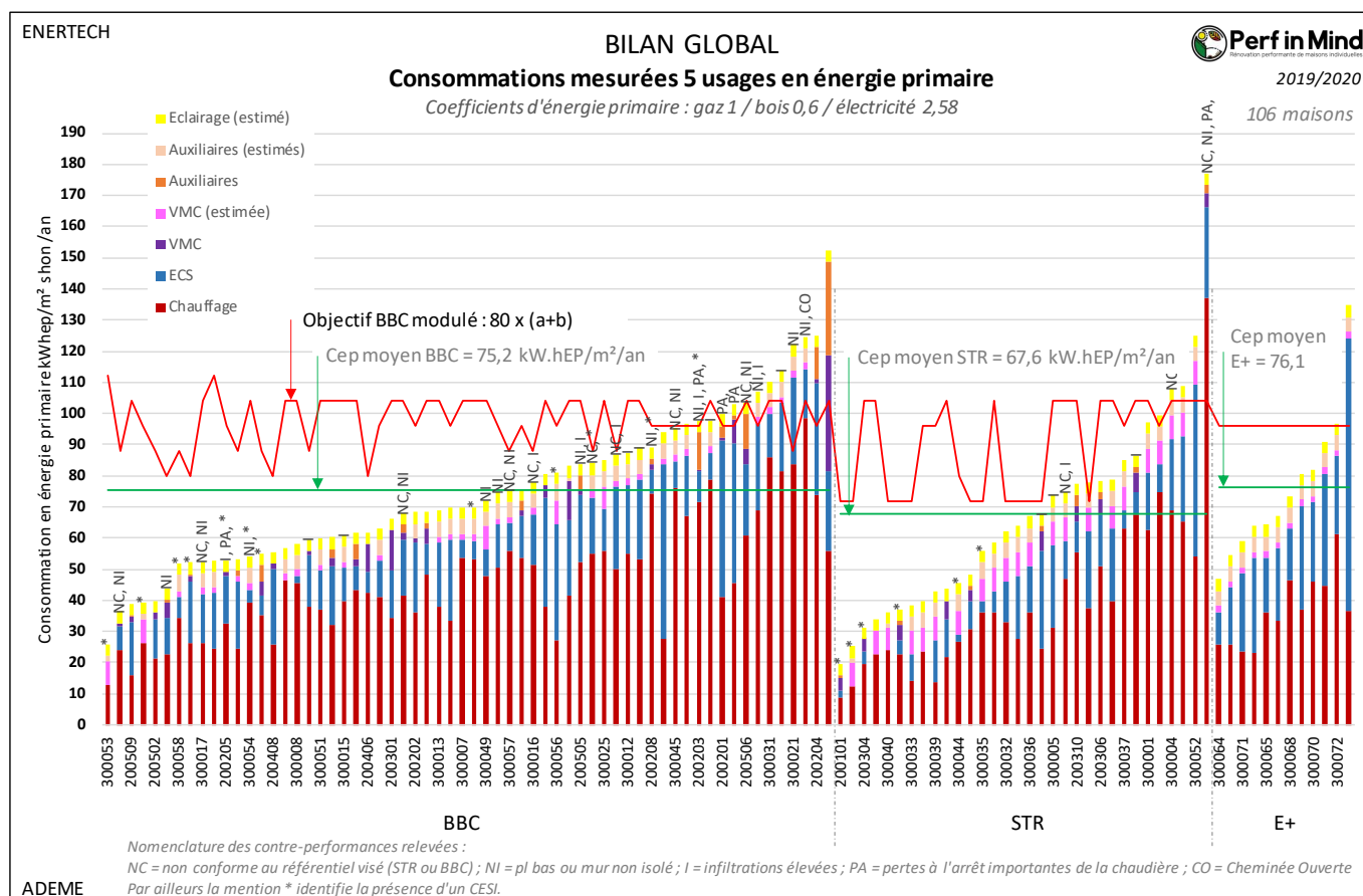
Figure 194 : Consommations mesurées sur les 5 postes du calcul réglementaire et comparaison aux objectifs BBC rénovation.
