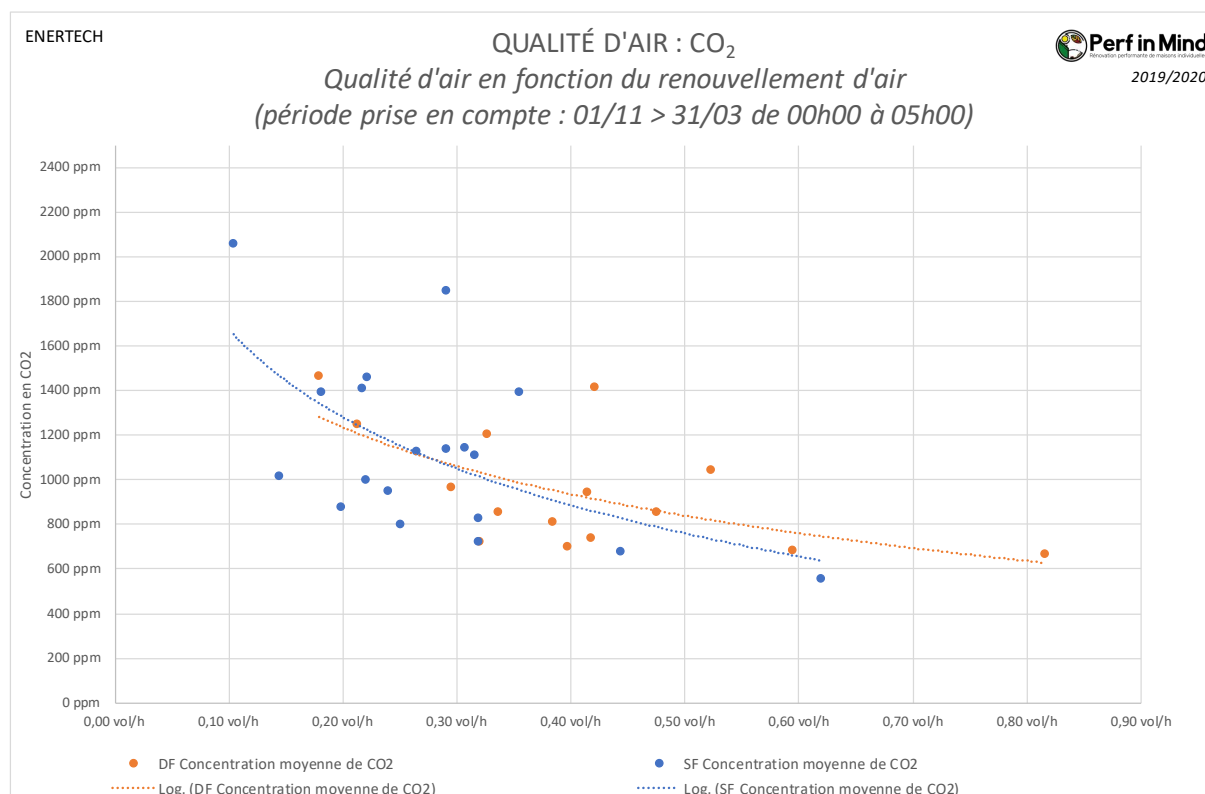
Figure 219 : Qualité d'air en fonction du taux de renouvellement d'air en taux de CO 2 moyen pendant la nuit.
