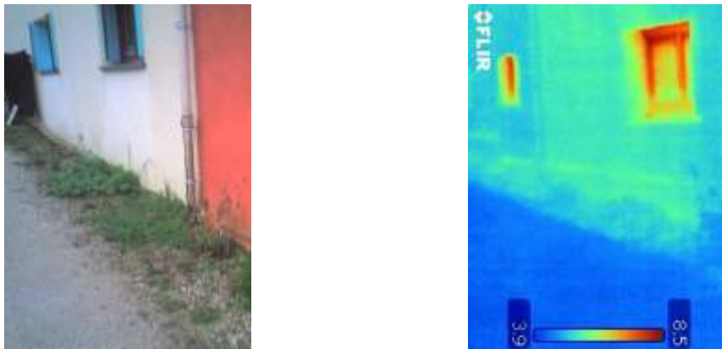
Figure 83 : Thermogramme de la liaison du mur avec le sol en présence d'une ITE enterrée.
