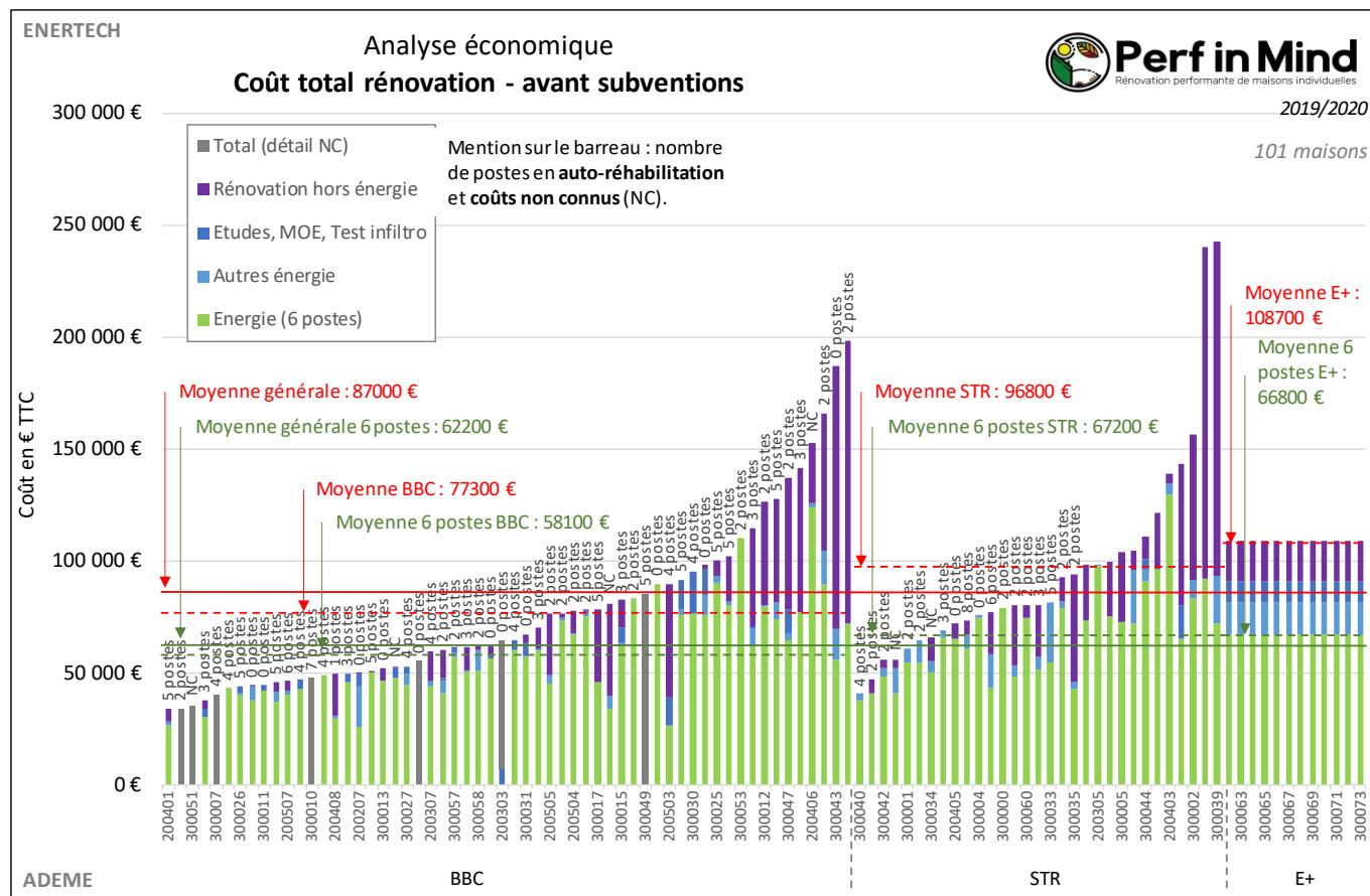
Figure 247 : Graphique des coûts totaux de rénovation.
