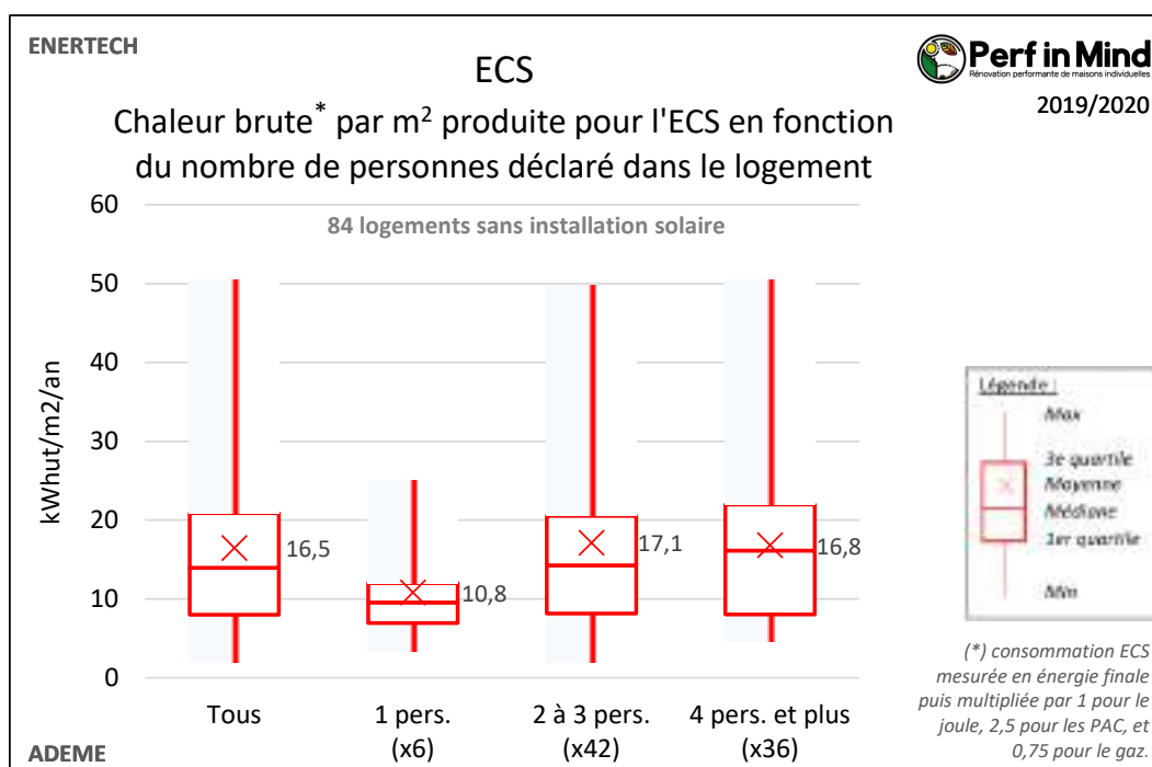
Figure 167 : Consommation de chaleur pour l'ECS par m 2 de surface shab.
