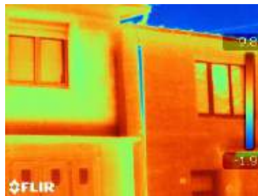
Figure 81 : Thermogramme de la façade d'une maison non isolée (à gauche) et de la maison suivie isolée par l'extérieur (à droite).
