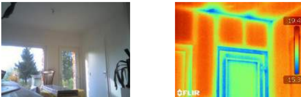
Figure 85 : Thermogramme des ponts thermiques d'ossature métallique traversant l'isolation intérieure.
