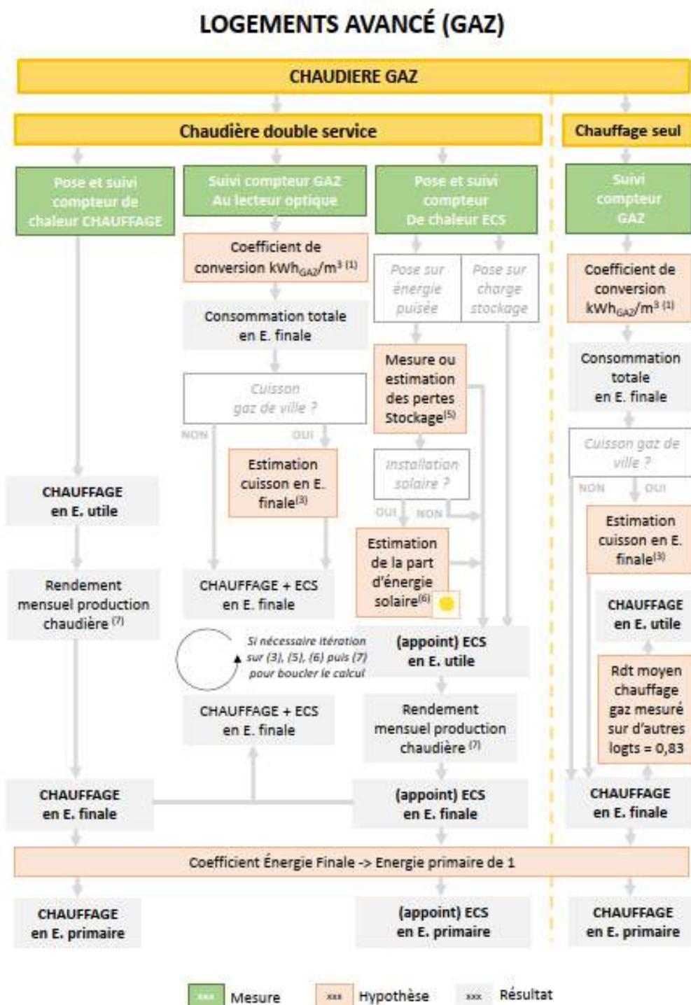
Figure 120 : Diagramme de traitement des données dans le cas des logements avancés au gaz (la mesure est indiquée en vert).
