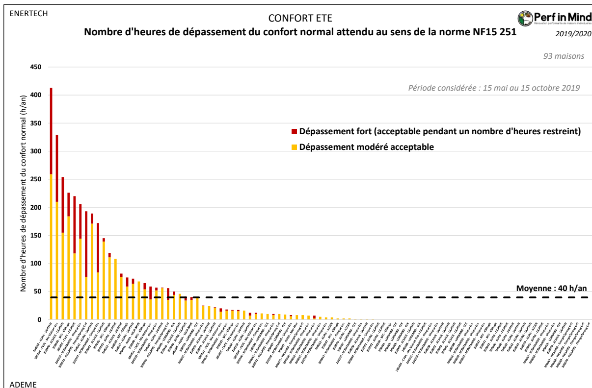
Figure 210 : Graphique du nombre d'heures de dépassement du confort normal attendu au sens de la norme NF 15 251.
