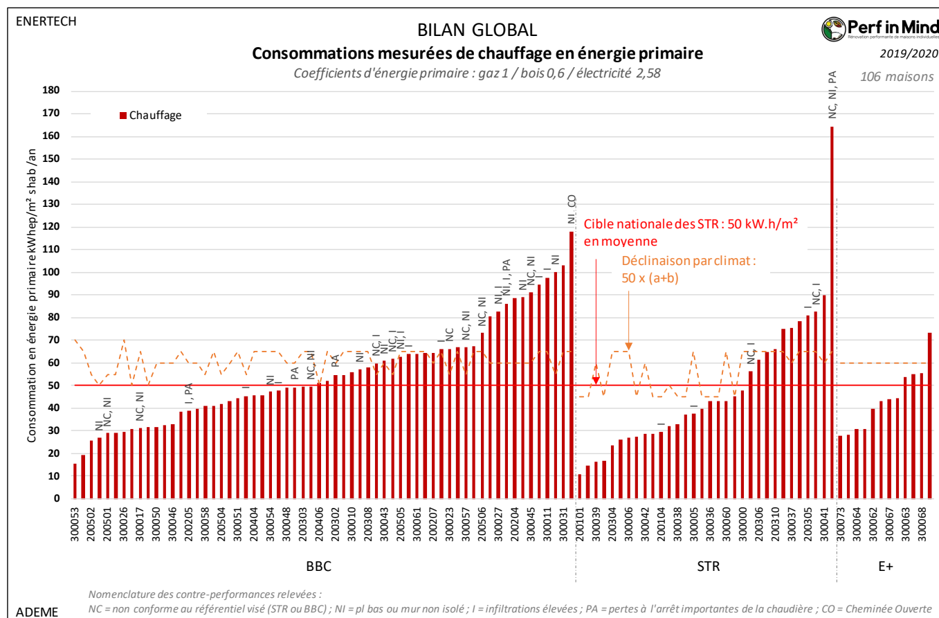
Figure 188 : Graphique des consommations de chauffage en énergie primaire. Comparaison aux objectifs des STR.
