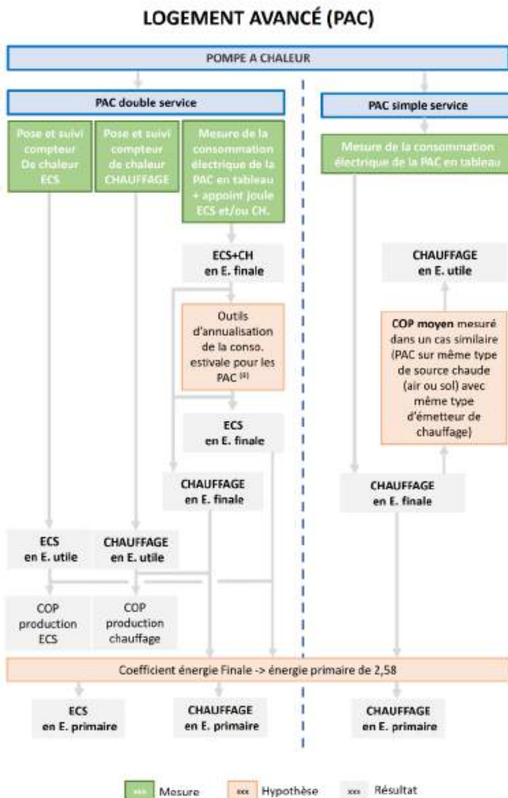
Figure 256 : Post-traitement de la mesure - logement avancé avec chauffage par pompe à chaleur.
