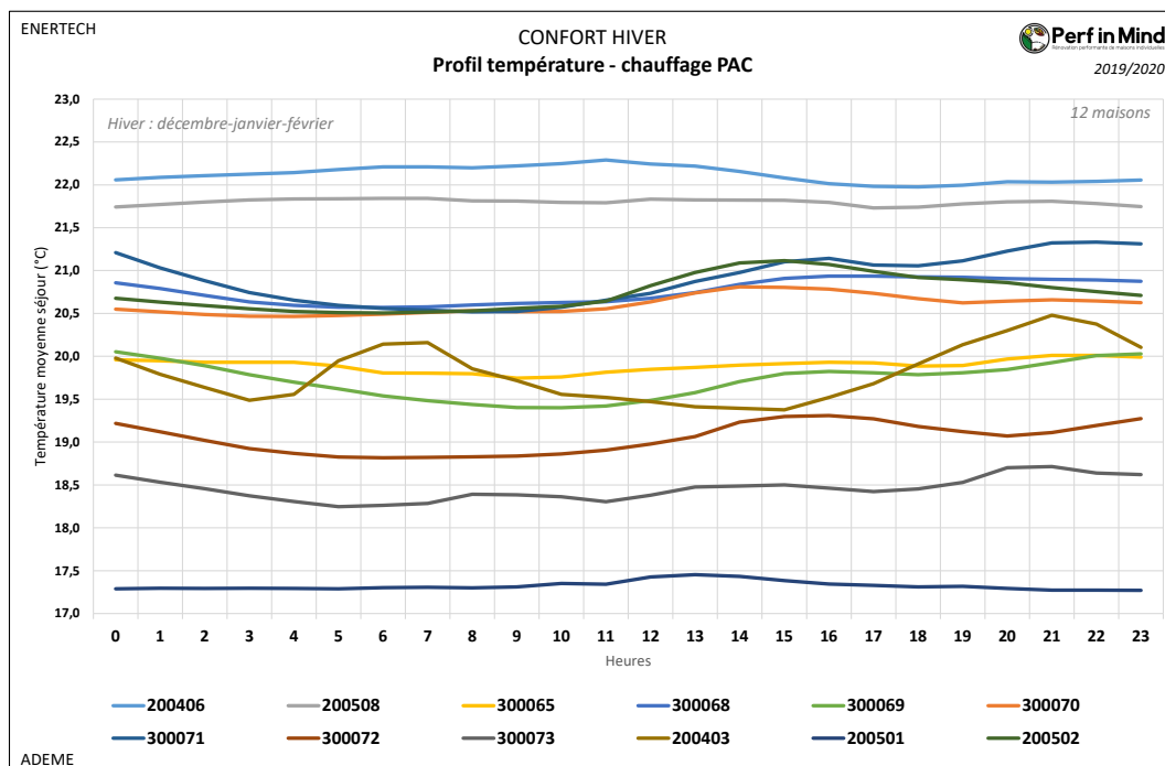
Figure 204 : Graphique des profils de température moyenne sur une journée pour les 12 maisons chauffées avec une pompe à chaleur.
