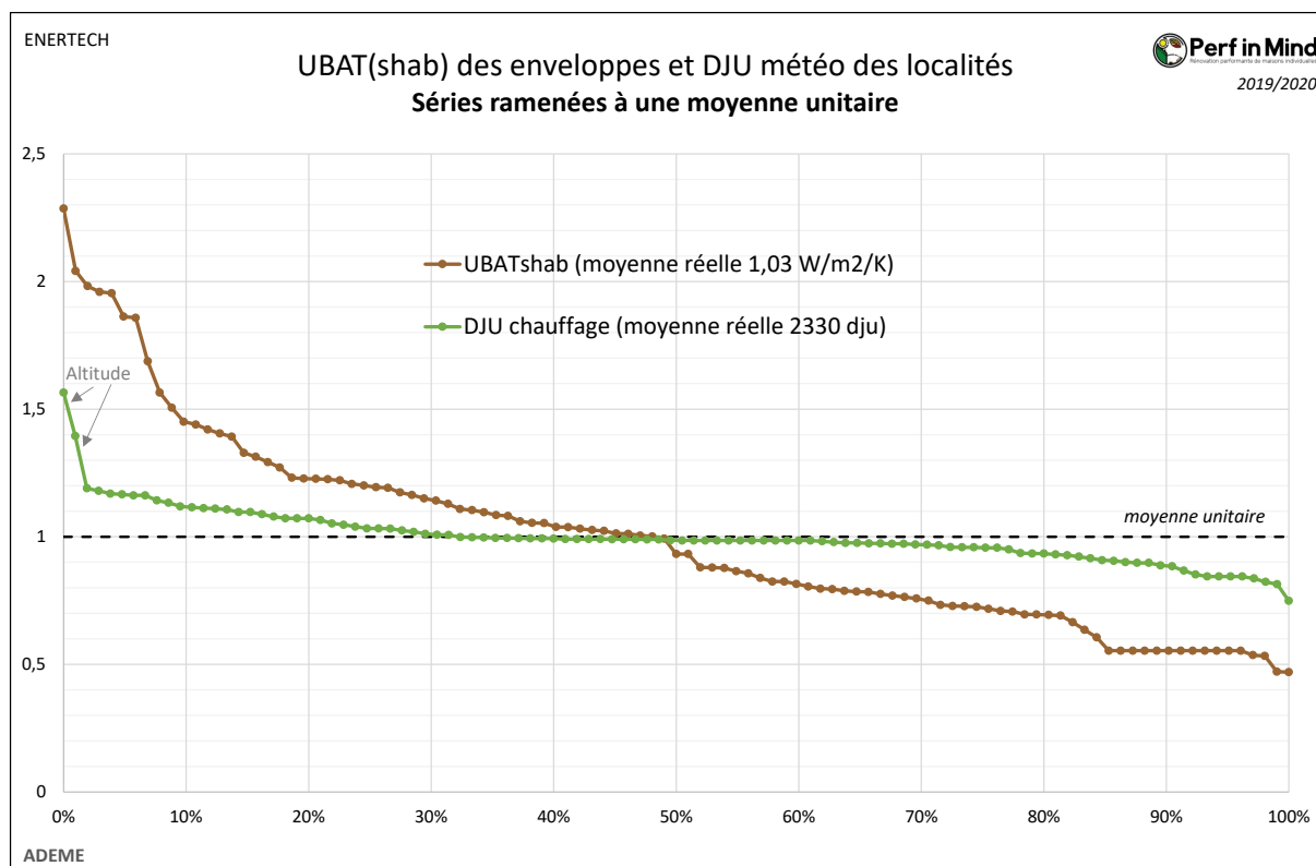
Figure 126 : Valeurs relatives des UBATshab et DJU rencontrées sur l'ensemble des projets.
