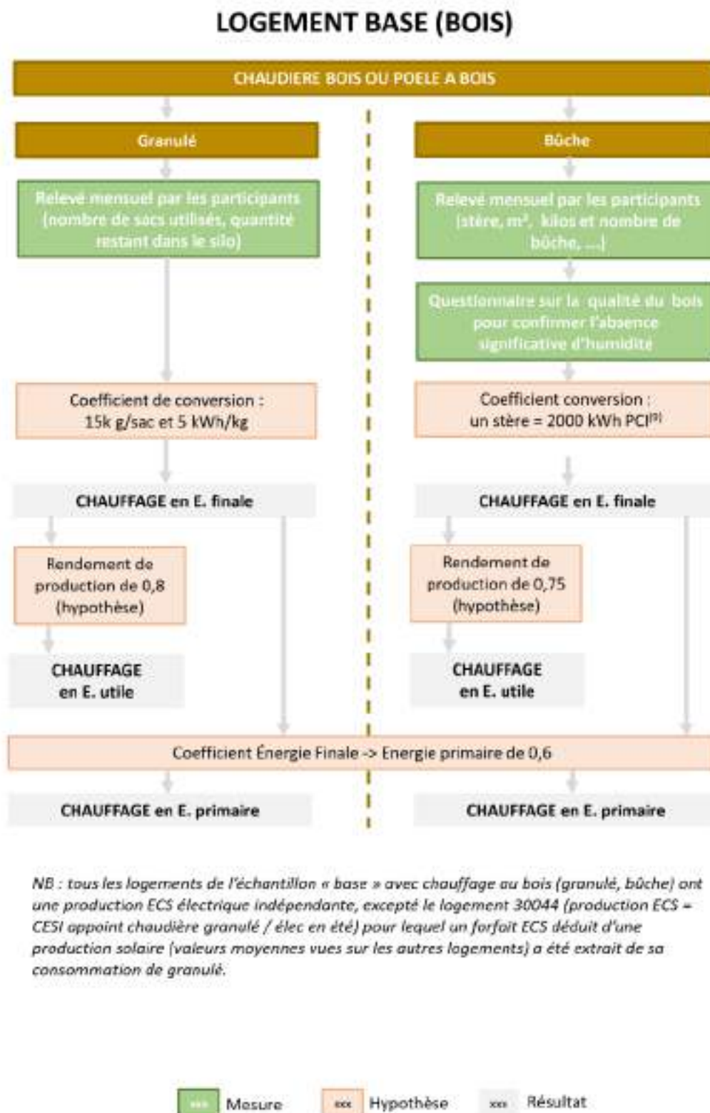
Figure 253 : Post-traitement de la mesure - logement base avec chauffage au bois.
