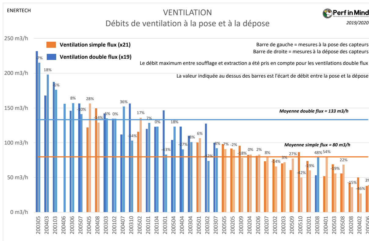
Figure 105 : Ventilation – Débits de ventilation mesurés à la pose et à la dépose
