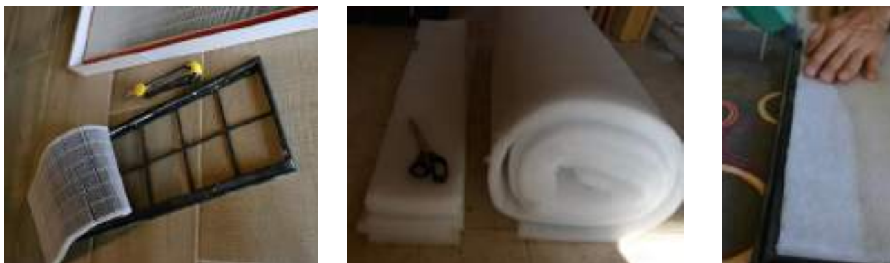
Figure 31 : Photos de la réalisation de filtres « maison » à partir d'un rouleau de médium filtrant (de type G4) : dépose du médium encrassé pour récupérer le cadre du filtre, découpe du médium filtrant neuf.
