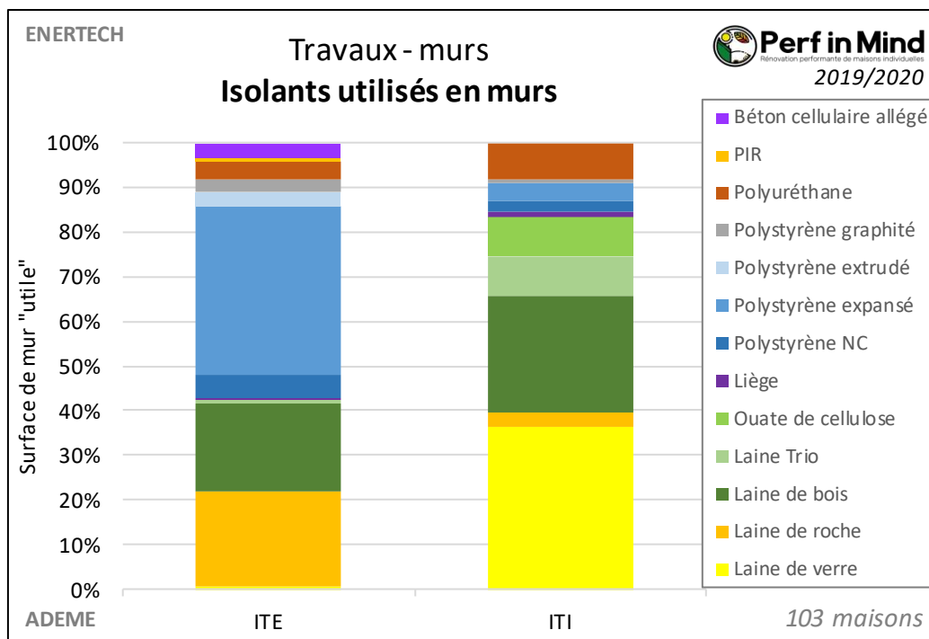
Figure 44 : Répartition des isolants utilisés en ITI et en ITE.
