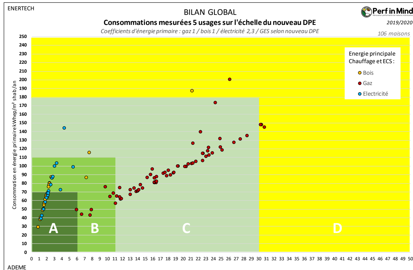
Figure 192 : Consommations mesurées de chauffage, ECS, auxiliaires (mesurés ou estimés) et éclairage (estimé, voir paragraphe suivant) et comparaison aux seuils énergétiques et GES du nouveau DPE. La couleur des marques indique l'énergie principale de chauffage et d'ECS.
