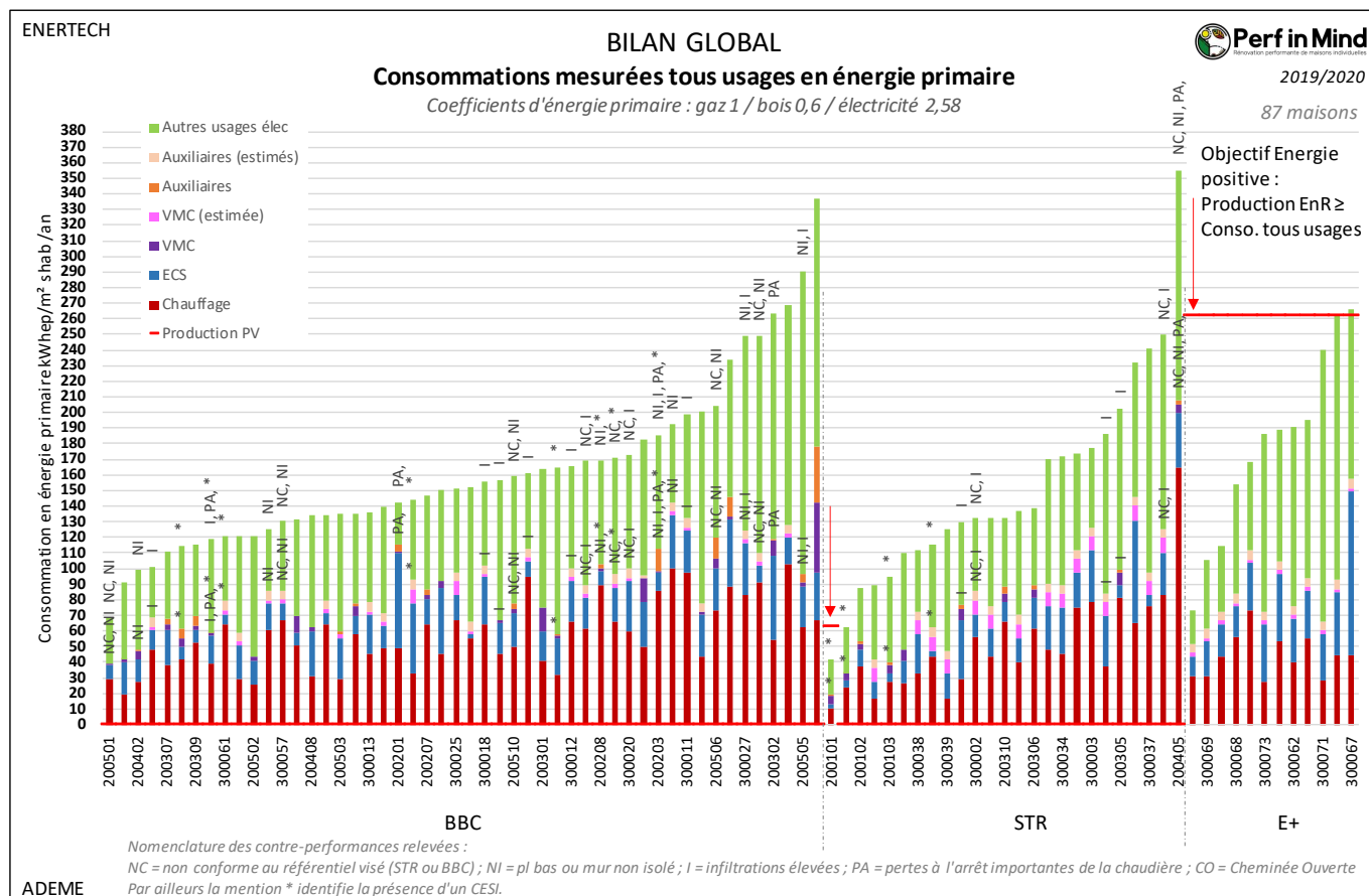
Figure 195 : Consommations mesurées tous usages et comparaison à l'objectif Energie positive.
