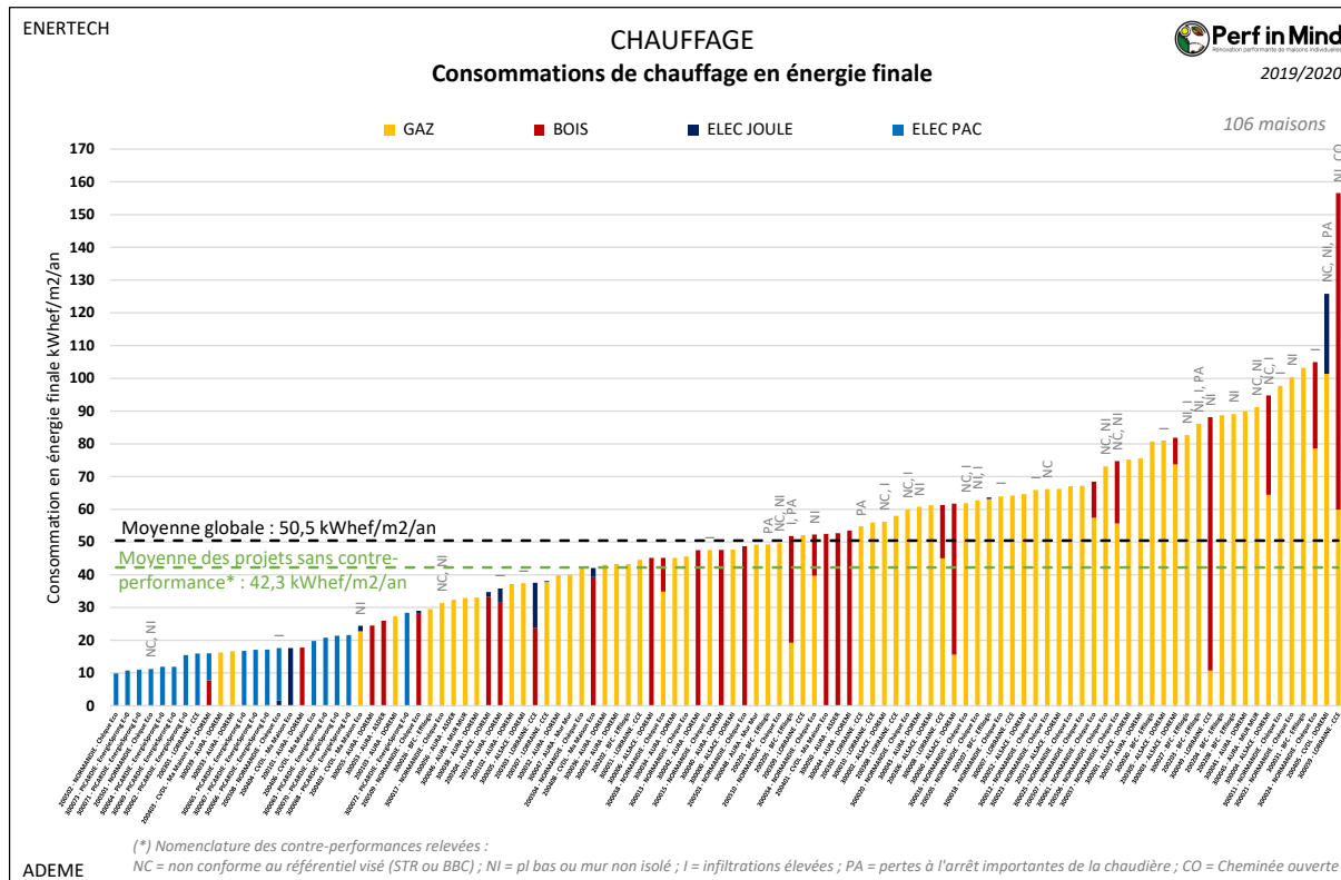
Figure 124 : Consommations de chauffage mesurées des projets en énergie finale.
