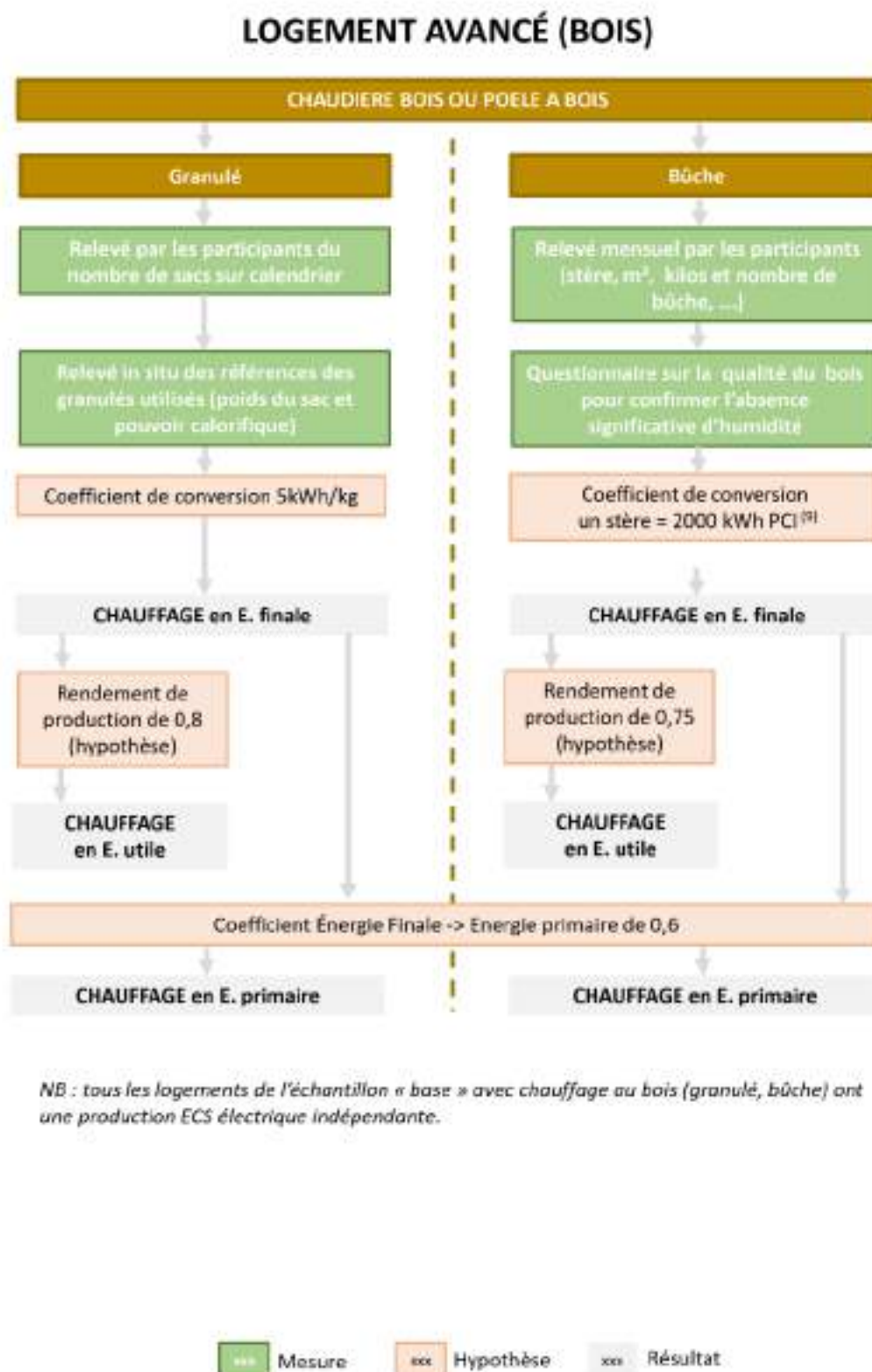
Figure 254 : Post-traitement de la mesure - logement avancé avec chauffage au bois.
