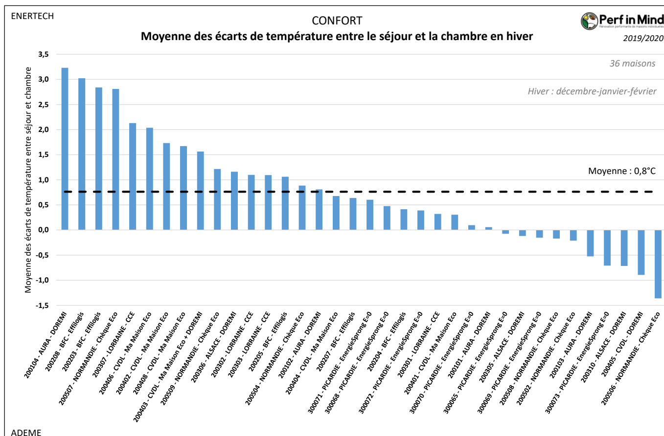
Figure 198 : Graphique de l'écart moyen de température entre le séjour et la chambre suivie le séjour en hiver.
