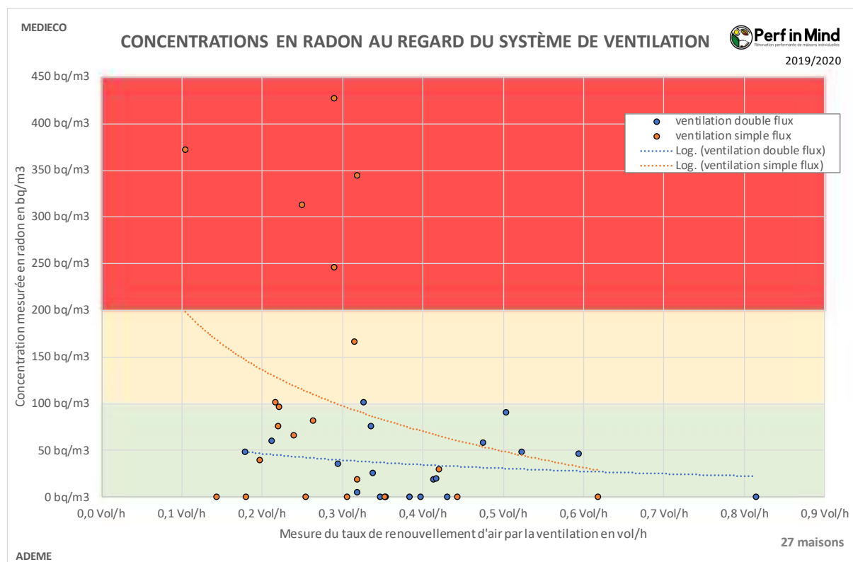
Figure 230 : Graphique des concentrations mesurées en radon en fonction du taux de renouvellement d'air mesuré.
