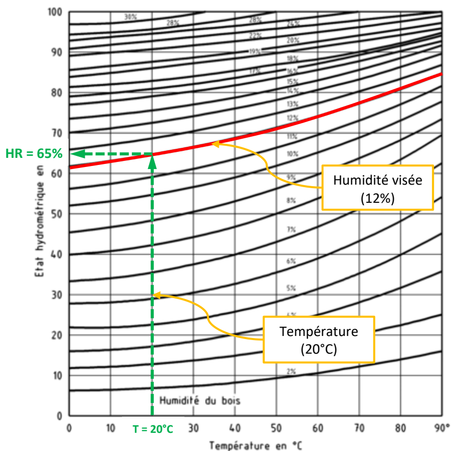
Figure 3 - Equilibre hygroscopique des bois mis en œuvre
