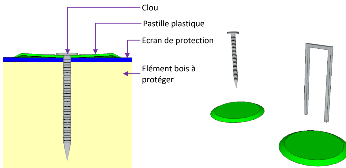
Figure 33 - Aperçu de fixations par agrafes ou clous avec pastilles
