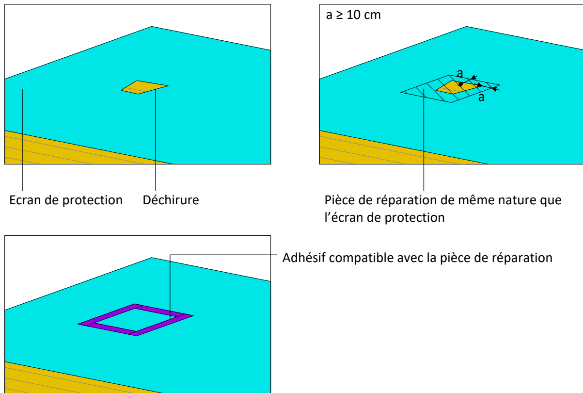
Figure 34 - Réparation d'une protection par empiècement (Source MATHIS)
