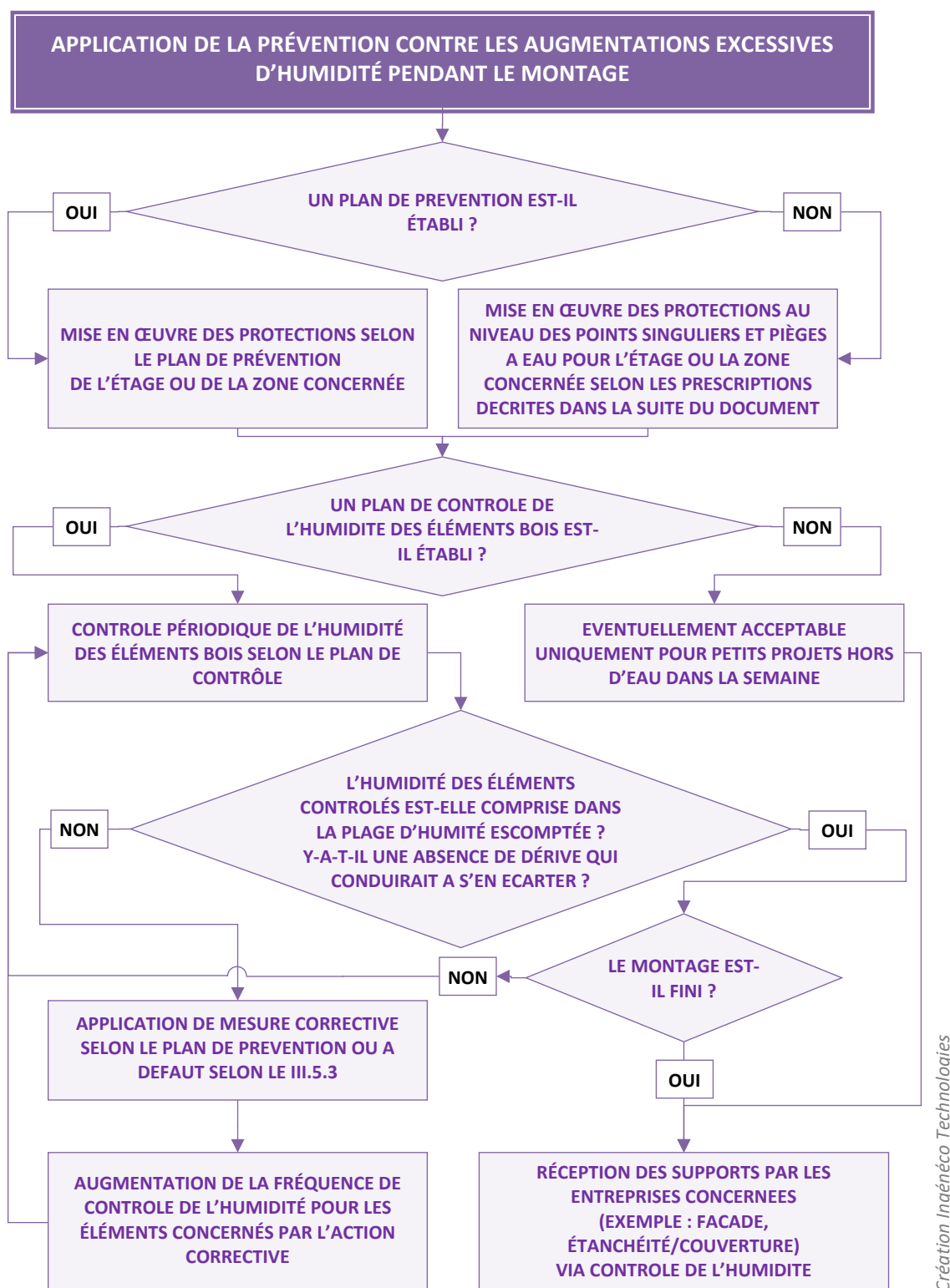
Figure 32 - application de la prévention contre les augmentations excessives d'humidité pendant le montage
