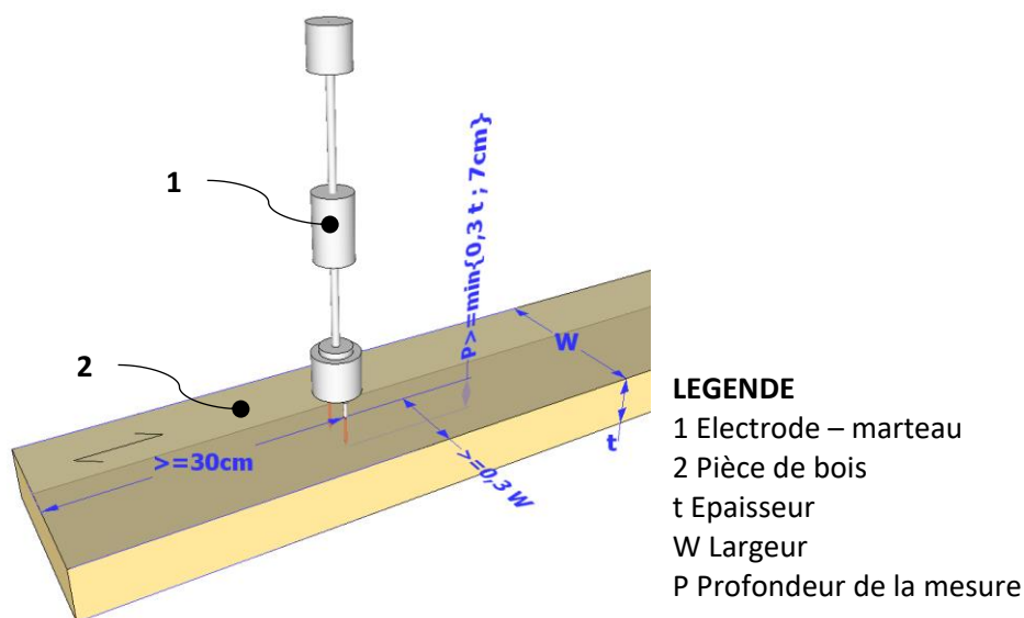
Figure 11 - Conditions minimales sur l'emplacement des mesures pour un humidimètre à pointe (issue de la figure 1 de la NF EN 13183-2)
