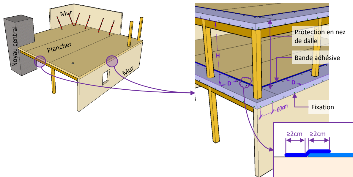
Figure 37 - Exemple de protection en nez de dalle
