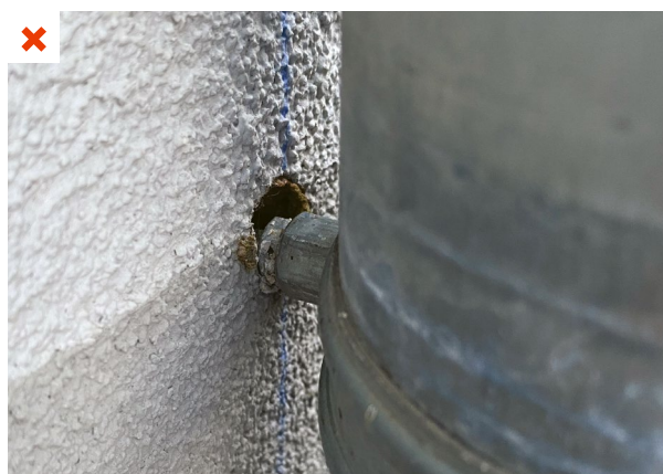
Les fixations des descentes d'eau pluviale traversant l'ITE ne sont pas adaptées. La tenue mécanique insuffisante entraîne une dégradation de l'isolant et la création d'un pont thermique. L'étanchéité à l'eau n'est plus assurée. ©AQC
