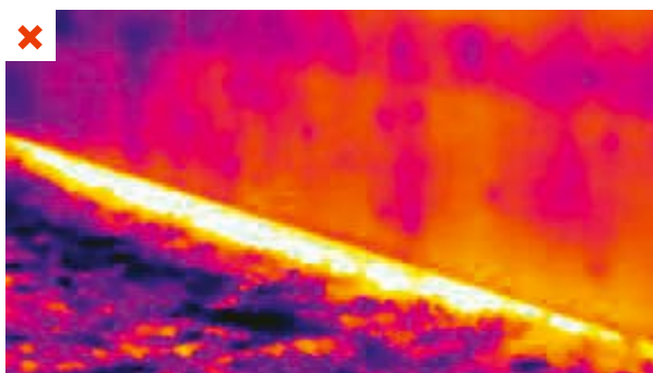
Le thermogramme permet de mettre en évidence les déperditions thermiques liées à l'absence d'isolation du soubassement. ©AQC
