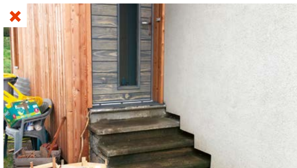
L'escalier en béton n'est pas désolidarisé de la façade isolée par l'extérieur et crée un pont thermique. ©AQC
