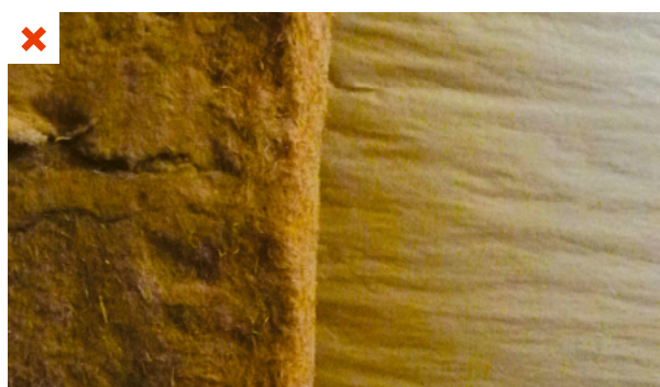
Les panneaux en fibre de bois sont appliqués en sous-face d'un pare-vapeur déjà en place. ©S.Courgey
