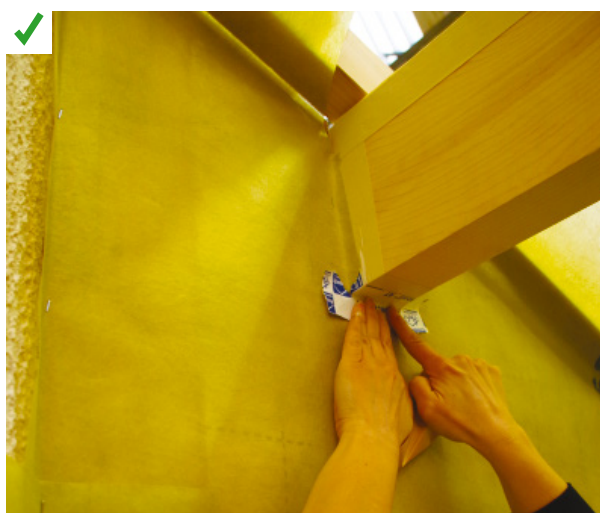
La membrane d'étanchéité à l'air est traversée par un élément de charpente. L'étanchéité à l'air de ce point singulier est traitée grâce à du ruban adhésif approprié qui permet de fixer la membrane sur le pourtour de la poutre. ©AQC
